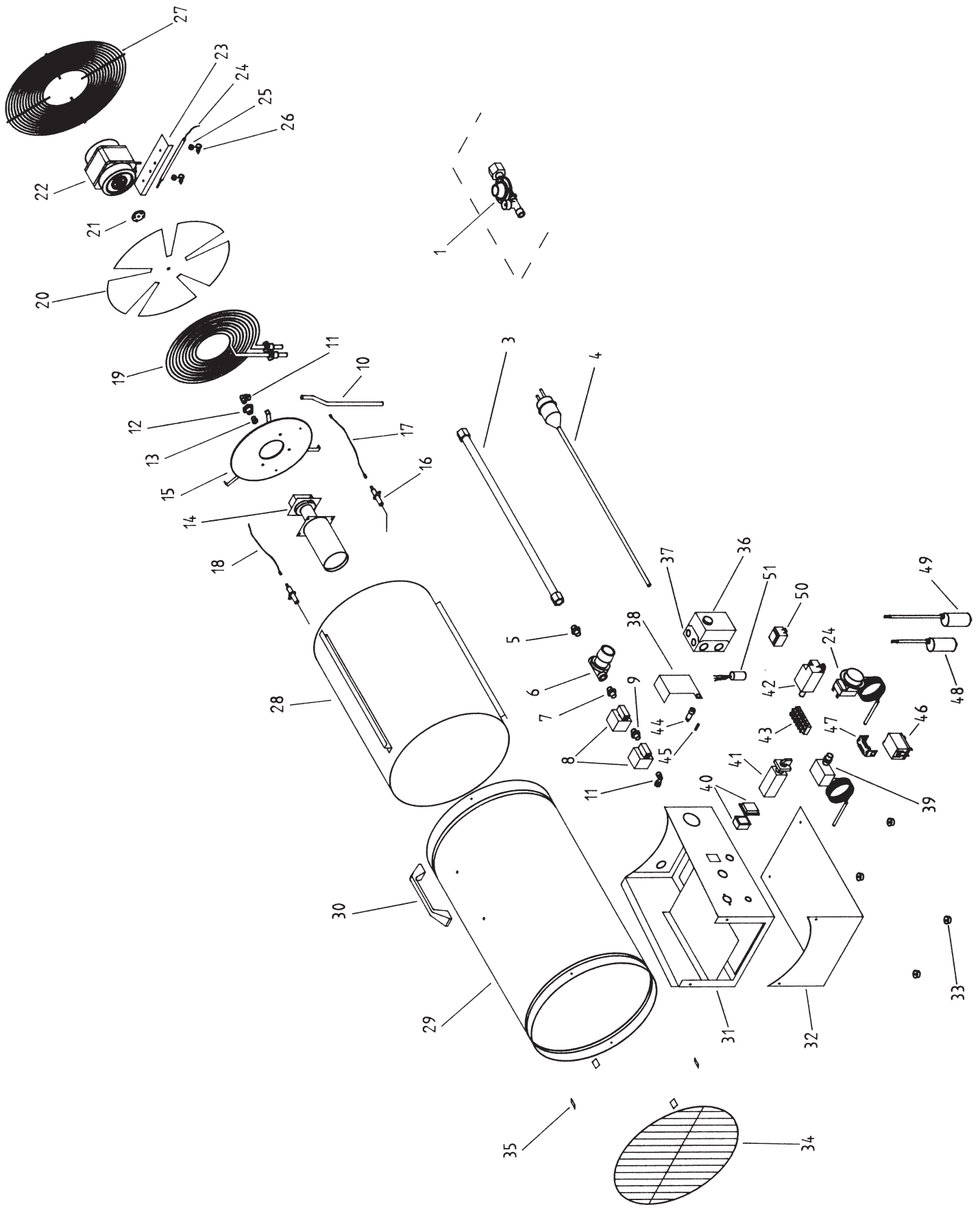
Explosionszeichnung GHE 26 TH (gültig ab 09/97)
